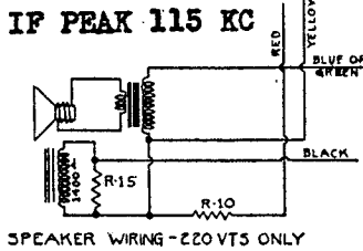
SCHEMATIC DIAGRAM PILOT MODEL 41 SUPER HET
